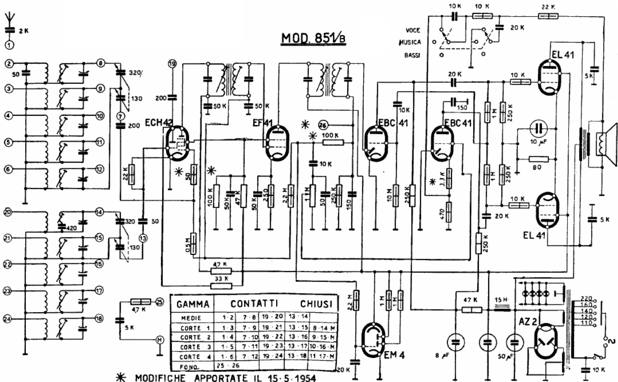
VEGA - Mod 581/B. Una gamma onde medie e quattro gamme onde corte. Media frequenza 470 kc/s. Potenza indistorta di uscita 15 watt. Consumo 80 watt.
